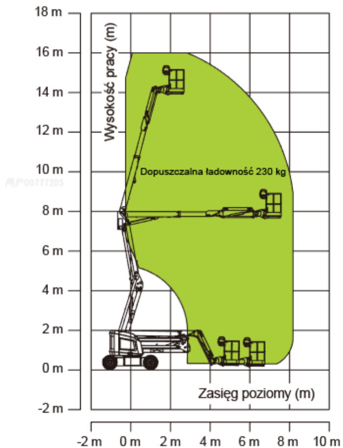
Rysunek 7-1 Zakres ruchu ZA14NJE-Li
