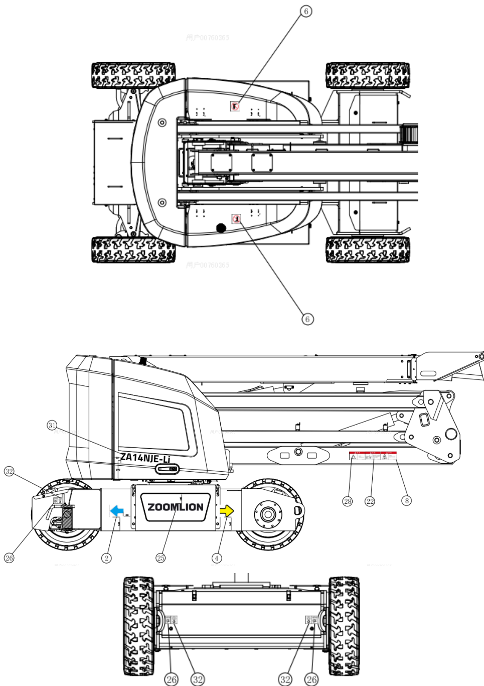
Rysunek 3-1 Położenie tabliczek (ciągły)
