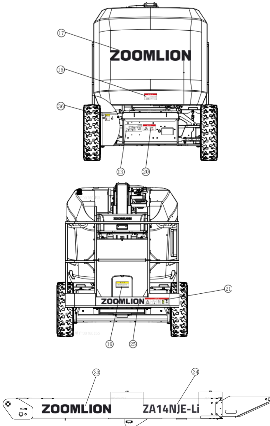
Rysunek 3-1 Położenie tabliczek (ciągły)
