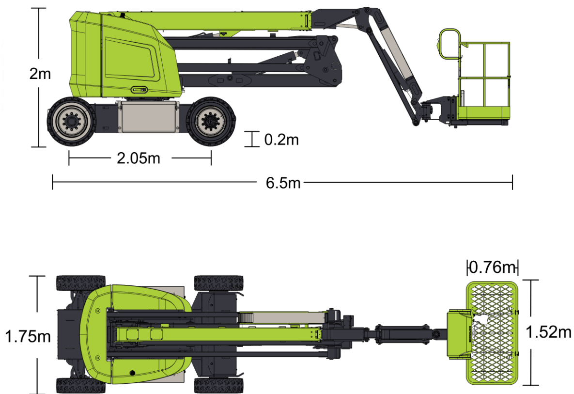
Rysunek 7-2 Wymiar ZA14NJE-Li w trybie transportowym
