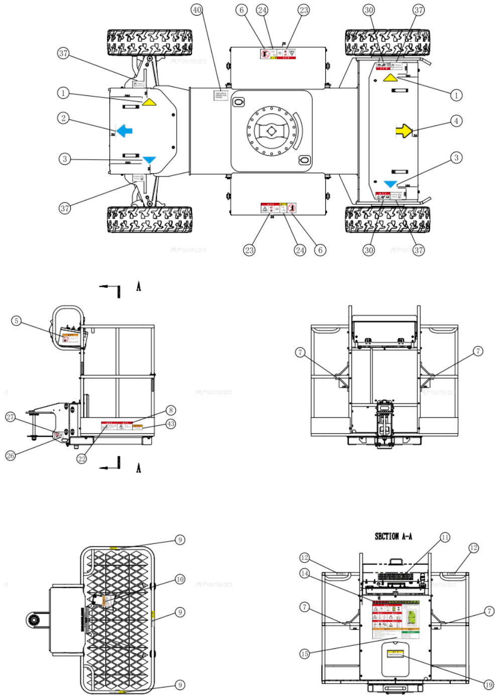
Rysunek 3-1 Położenie tabliczek
